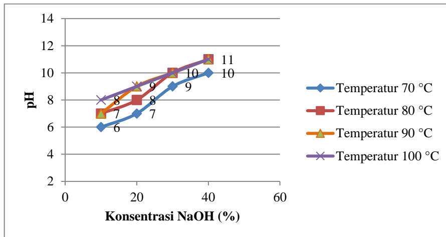
Grafik 2. Hubungan Antara Konsentrasi NaOH dan pH Terhadap Temperatur
