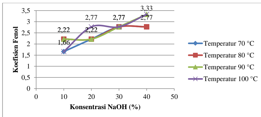
Grafik 1. Hubungan Antara Konsentrasi NaOH dan Koefisien Fenol Terhadap Temperatur
