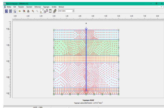
Gambar 5. Tegangan Efektif
