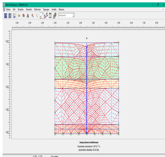
Gambar 3. Jaring Terdeformasi
