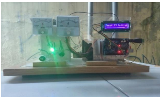
Gambar 16. Hasil Pengujian Sensor Suhu
