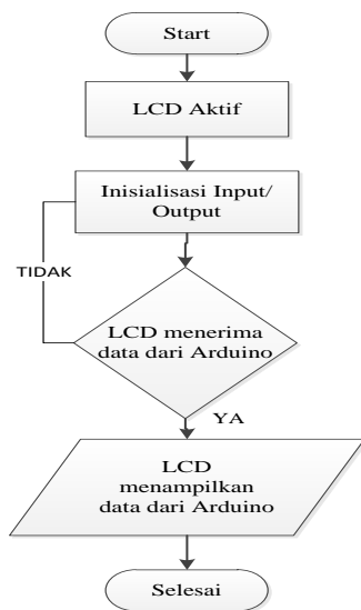
Gambar 4. Diagram Alir Mesin Pendingin dari LCD
