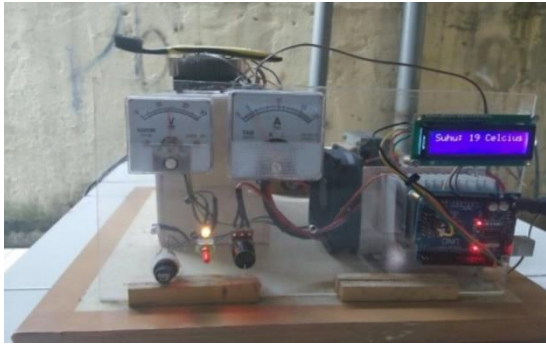
Gambar 14. Rangkaian Keseluruhan
