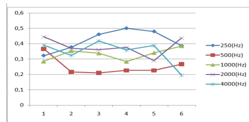
Gambar 2. Grafik Frekuensi terhadap koefisien serap bunyi pada variasi 20%
