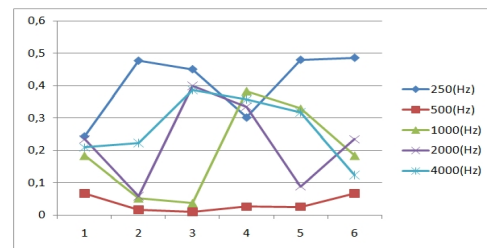
Gambar 1. Grafik Frekuensi terhadap koefisien serap bunyi pada variasi 0%
