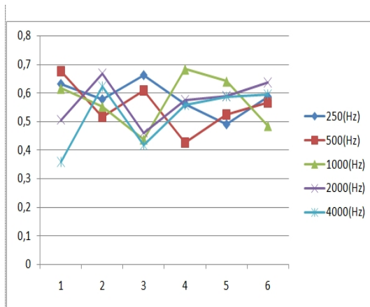
Gambar 3. Grafik Frekuensi terhadap koefisien serap bunyi pada variasi 30%
