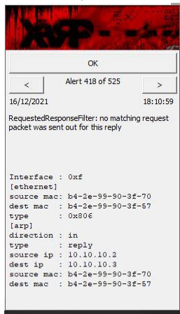
Gambar 6 Menampilkan Notifikasi (Alert)
