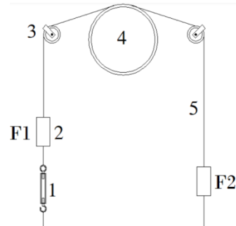
Gambar 1. Skema pengukuran torsi
