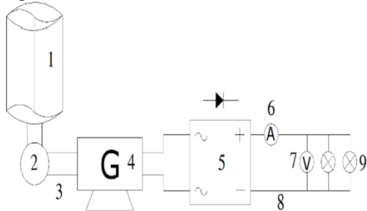
Gambar 2. Skema pengukuran daya generator
