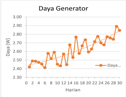
Gambar 11. Pengujian Daya generator
