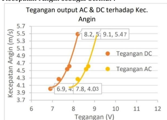
Gambar 8. Grafik antara Tegangan dan Kecepatan Angin
