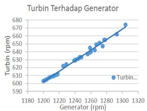
Gambar 7. Putaran turbin terhadap putaran generator
