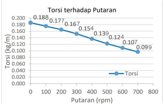
Gambar 10. Grafik Torsi terhadap Putaran
