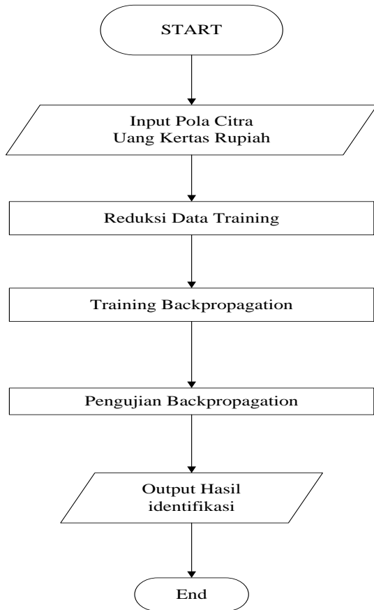
Gambar 6. Flowchart Sistem aplikasi deteksi keaslian uang dengan metode backpropagation
