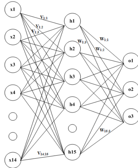
Gambar 5. Arsitektur Jaringan Backpropagation Identifikasi Keaslian Uang Tipe Nominal Uang
