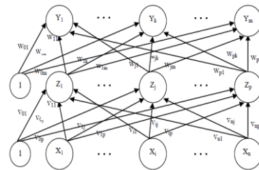
Gambar 1. Arsitektur jaringan backpropagation dengan satu lapisan tersembunyi (Drs. Jong Jek Siang, 2006)
