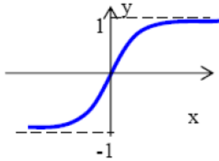
Gambar 2. Fungsi Aktivasi Sigmoid Bipolar (Diyah Puspitaaningrum, 2006)
