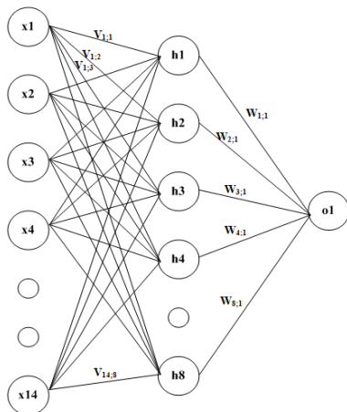
Gambar 4. Arsitektur Jaringan backpropagation Identifikasi Keaslian Uang Tipe Status uang
