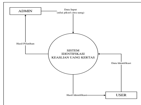
Gambar 3. Diagram Konteks
