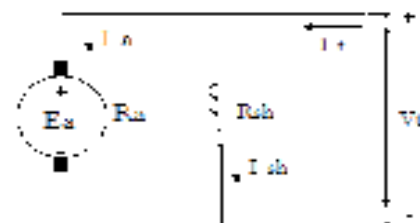
Gambar 2. Rangkaian listrik Motor DC Shunt
