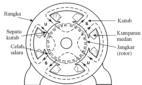
Gambar 1. Bagian Komponen Motor DC Shunt
