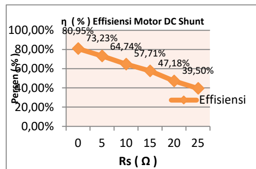
Gambar 7. Pengaruh penambahan tahanan Rs terhadap efisiensi motor DC shunt
