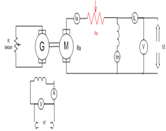
Gambar 6. Rangkaian motor DCshunt dengan penambahan tahanan R_s dan dengan beban generator
