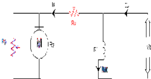
Gambar 5. Rangkaian motor DCshunt dengan R_s terhubung seri dan R_p terhubung paralel terhadap tahanan jangkar motor
