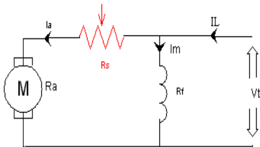
Gambar 4. Rangkaian motor DCshunt dengan tahanan R_s terhubung seri dengan tahanan jangkar motor DC shunt
