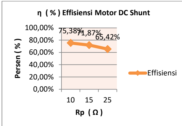
Gambar8. Pengaruh penambahan tahanan R_s dan R_p terhadap efisiensi motor dc
