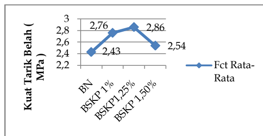
Gambar 4. Grafik Persentase nilai kuat tarik belah beton pada umur 28 hari.
