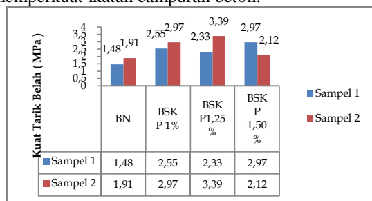
Gambar 3. Persentase nilai kuat tarik belah beton pada umur 28 hari.
