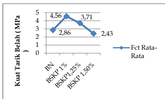
Gambar2. Grafik Persentase nilai kuat tarik belah beton pada umur 7 hari.
