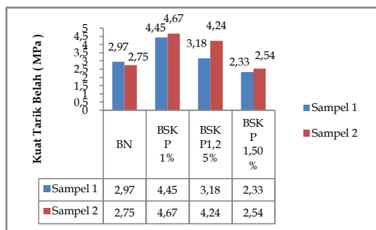
Gambar1. Persentase nilai kuat tarik belah beton pada umur 7 hari.
