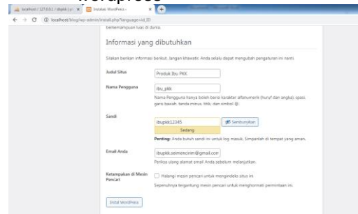
Gambar 5. Isi Informasi
