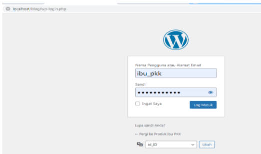
Gambar 7. Login
