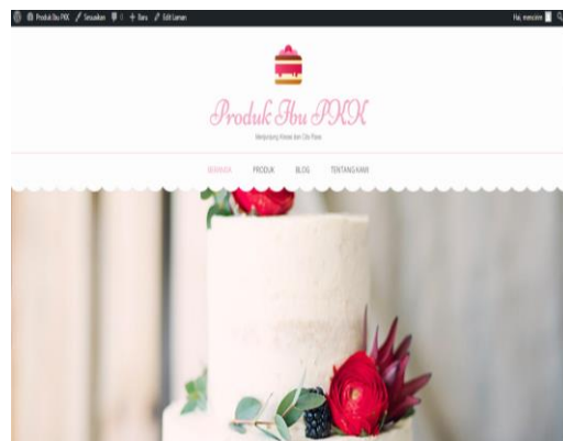
Gambar 17. Tampilan Webiste
