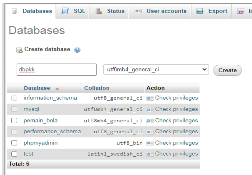
Gambar 1. Membuat Databases
