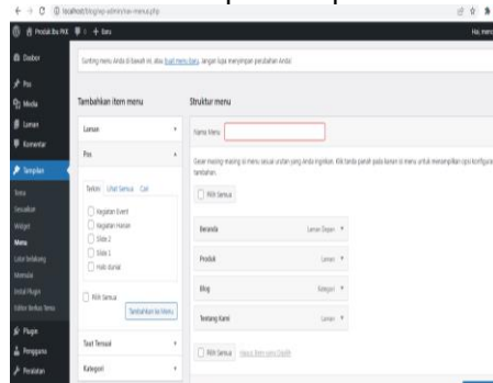
Gambar 12. Tampilan Menu
