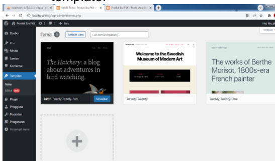
Gambar 9. Tampilan Tema
